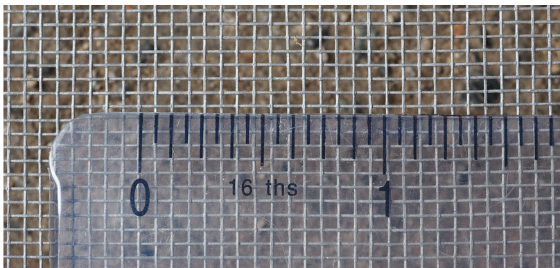
RESPIRADEROS APROBADOS POR WUI (1/16 - 1/8")
